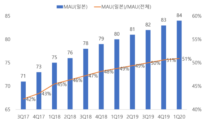
그림 5-4. 라인 MAU
