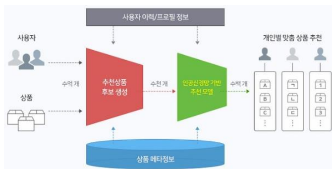
그림 3-21. AiTEMS 개요
